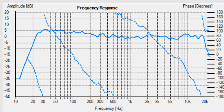
Kmitočtová charakteristika
